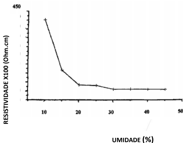
Fig. 01 – Variação da Resistividade Elétrica com o Teor de Umidade.
