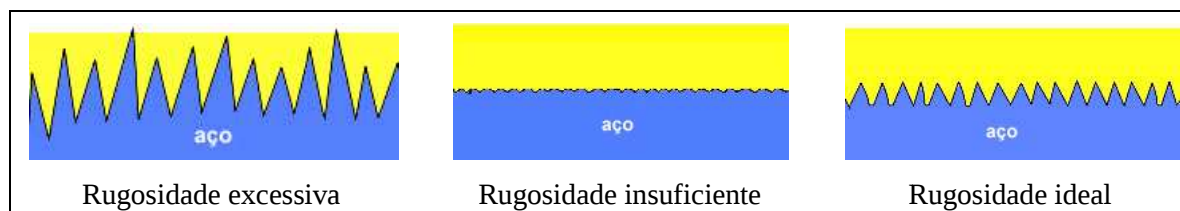
Figura 5 - Comparação entre perfis de rugosidade
