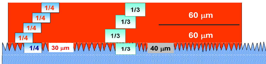
Figura 6 - Perfis de rugosidade para atender ao requisito de 1/4 a 1/3 da espessura total do esquema de pintura ( 120\ \mu\text{m} ), previsto na ABNT NBR 7348 [5].
