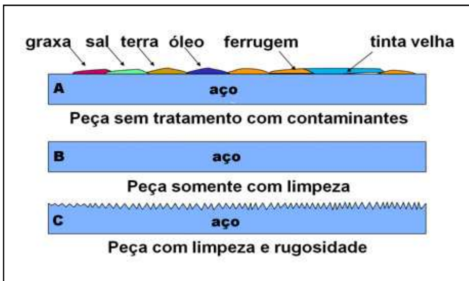
Figura 2 - Ilustração de aspectos superficiais de substratos de aço.
