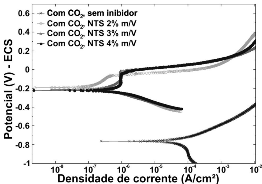
Figura 1 - Curvas de polarização anódica do aço 1020 em soluções de SSP + NaCl 3% m.V -1 sem inibidor e SSP + NaCl 3% m.V -1 + NTS 2%, 3% e 4% m.V -1 , com borbulhamento de gás CO 2 , pH final 7.
