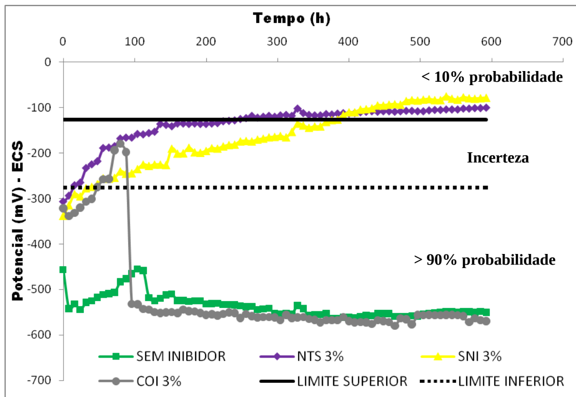
Figura 4 - Resultados de ensaios de potencial de corrosão em função do tempo realizados em SSP + NaCl 3% m.V -1 sem inibidor e na presença de todos os inibidores testados, na concentração 3% m.V -1 , após o borbulhamento de \text{CO}_2 .
