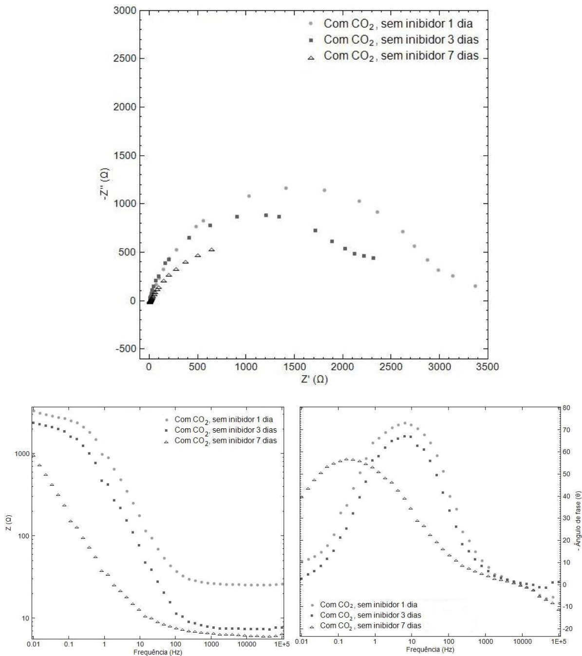
Figura 5 - Diagramas de Nyquist (superior), Módulo de Bode (esquerda) e Ângulo de fase de Bode (direita) para o eletrodo de aço 1020 imerso em solução sintética de poros, com NaCl, sem inibidor, após borbulhamento de \text{CO}_2 após 1, 3 e 7 dias de imersão.
