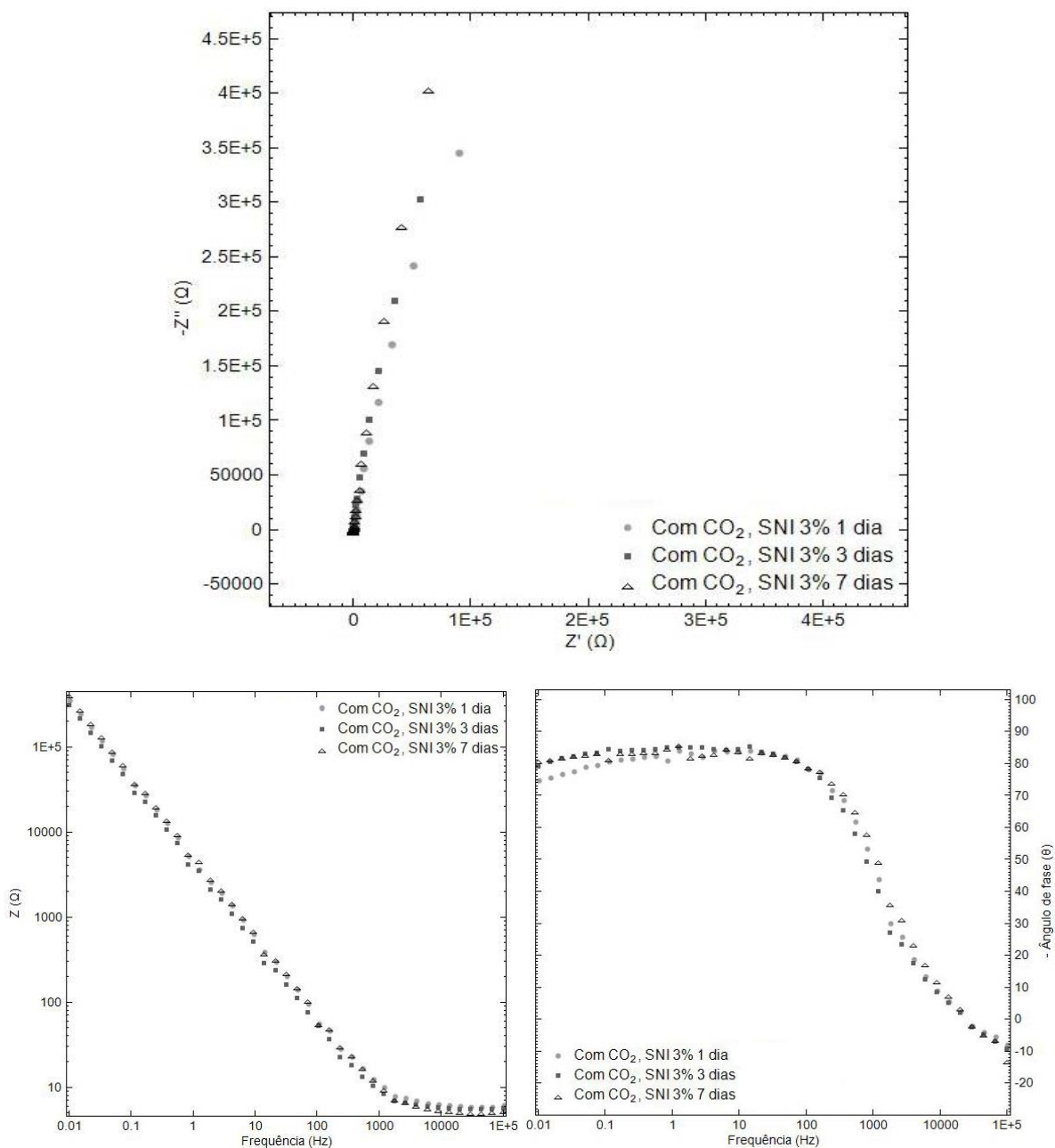
Figura 9 - Diagramas de Nyquist (superior), Módulo de Bode (esquerda) e Ângulo de fase de Bode (direita) para o eletrodo de aço 1020 imerso em solução sintética de poros com NaCl, contendo SNI 3% m.V -1 , após borbulhamento de CO 2 , com 1, 3 e 7 dias de imersão.
