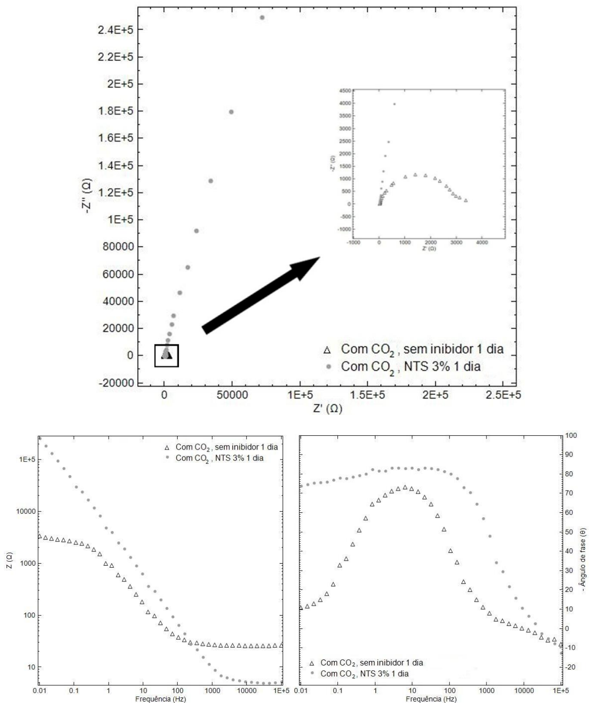
Figura 6 - Diagramas de Nyquist (superior), Módulo de Bode (esquerda) e Ângulo de fase de Bode (direita) para o eletrodo de aço 1020 imerso em SSP com NaCl, NTS 3% m.V -1 e em SSP sem inibidor, com 1 dia de imersão, ambos após borbulhamento de CO 2 .
