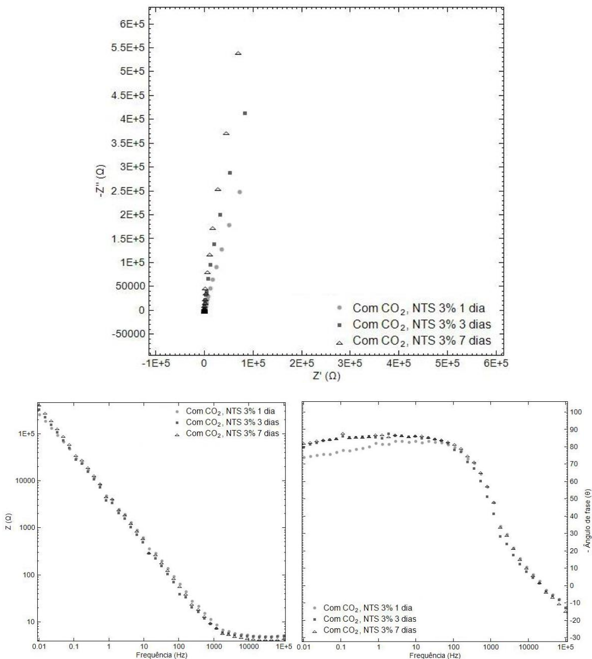
Figura 7 - Diagramas de Nyquist (superior), Módulo de Bode (esquerda) e Ângulo de fase de Bode (direita) para o eletrodo de aço 1020 imerso em solução sintética de poros com NaCl, contendo NTS 3% m.V -1 , após borbulhamento de CO 2 , com 1, 3 e 7 dias de imersão.
