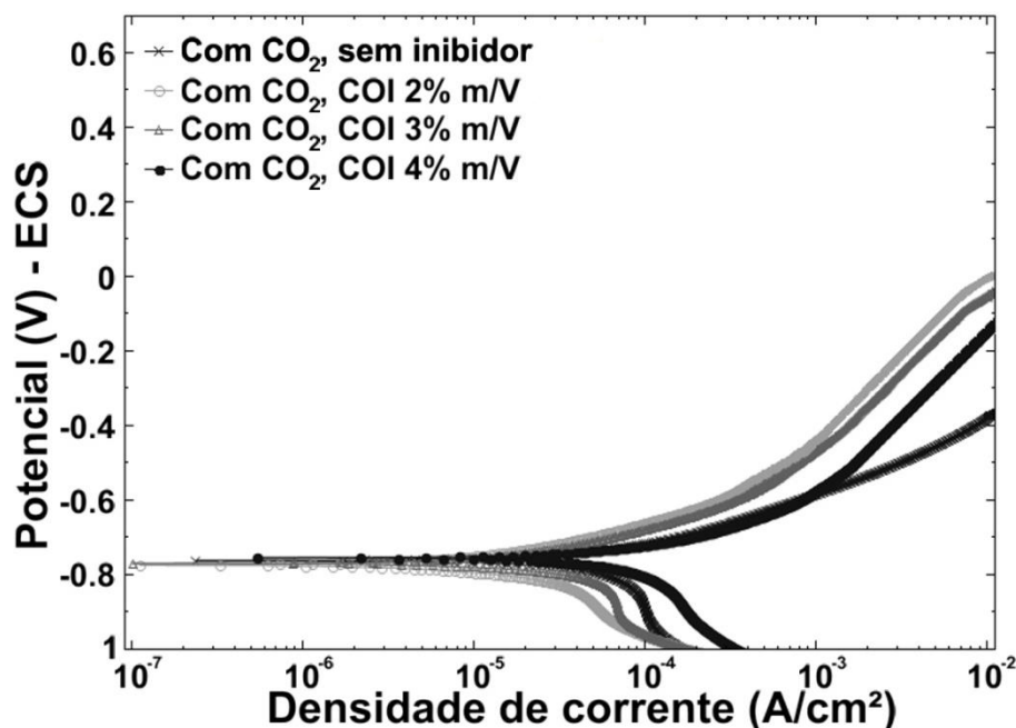
Figura 3 - Curvas de polarização anódica do aço 1020 em soluções de SSP + NaCl 3% m.V -1 sem inibidor e SSP + NaCl 3% m.V -1 + COI 2%, 3% e 4% m.V -1 , com borbulhamento de gás CO 2 , pH final 7.
