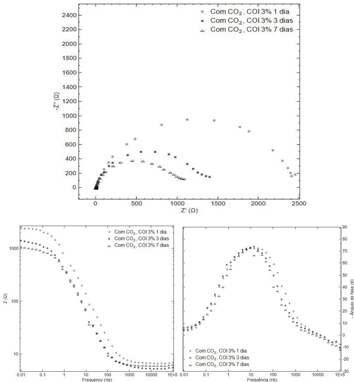
Figura 11 - Diagramas de Nyquist (superior), Módulo de Bode (esquerda) e Ângulo de fase de Bode (direita) para o eletrodo de aço 1020 imerso em solução sintética de poros com \text{NaCl} , contendo \text{COI} 3% \text{m.V}^{-1} , após borbulhamento de \text{CO}_2 , com 1, 3 e 7 dias de imersão.
