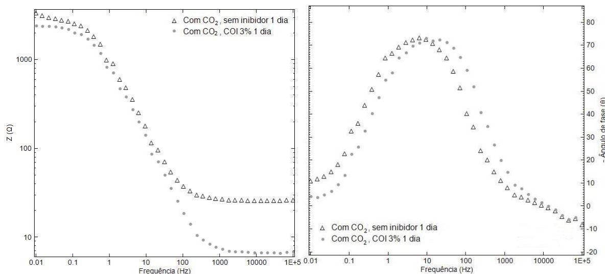
Figura 10 - Diagramas de Nyquist (superior), Módulo de Bode (esquerda) e Ângulo de fase de Bode (direita) para o eletrodo de aço 1020 imerso em SSP com NaCl e COI 3% m.V -1 e em SSP sem inibidor, com 1 dia de imersão, ambos após borbulhamento de CO 2 .
