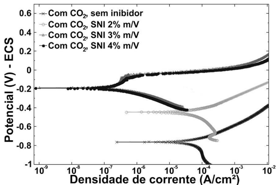
Figura 2 - Curvas de polarização anódica do aço 1020 em soluções de SSP + NaCl 3% m.V -1 sem inibidor e SSP + NaCl 3% m.V -1 + SNI 2%, 3% e 4% m.V -1 , com borbulhamento de gás CO 2 , pH final 7.
