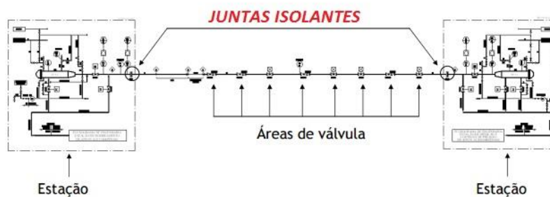
Figura 1 - Esquemático de Instalação das Juntas de Isolamento em um Sistema de Proteção Catódica
