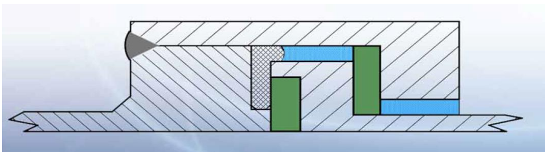
Figura 6 - Selo de Vedação do tipo Retangular
