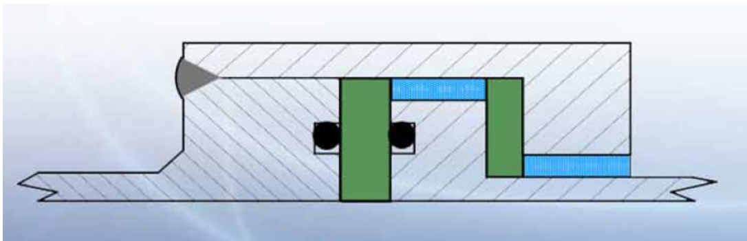
Figura 5 - Selo de Vedação do tipo O-Ring
