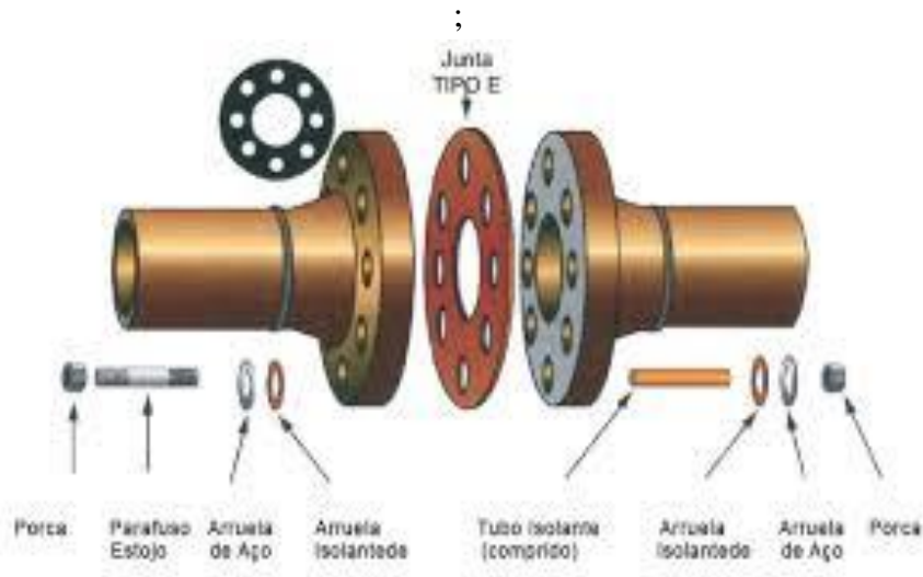
Figura 2 - Junta de Isolamento Elétrico Convencional entre flanges
