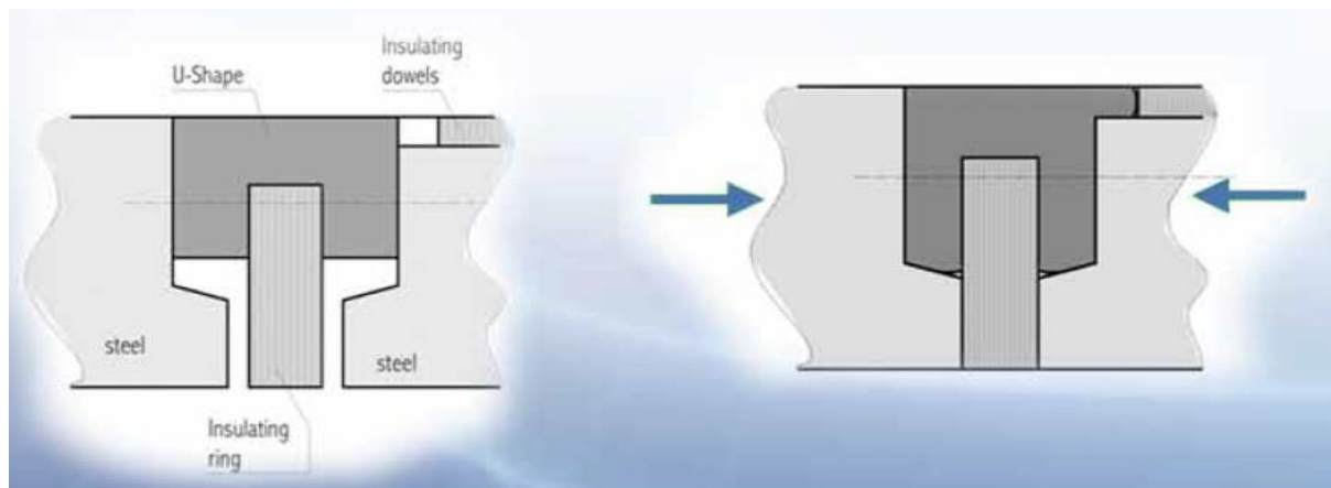
Figura 12 - Sistema de Vedação do tipo Formato em "U" antes e depois da montagem
