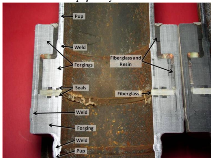
Figura 4: Exemplo de junta de isolamento elétrico monobloco cortada
