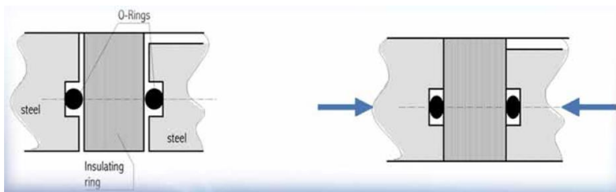
Figura 11 - Esquemático de deformação / compressão do Selo O-Ring
