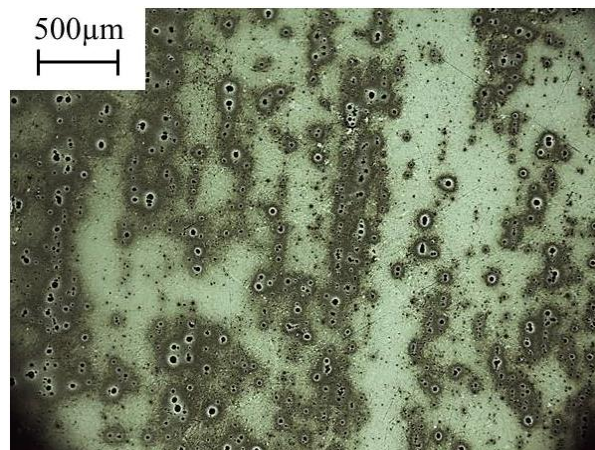
Figura 6- Corrosão localizada na liga AA2198-T851 associada às presença de partículas contituíntes micrométricas na superfície da liga.
