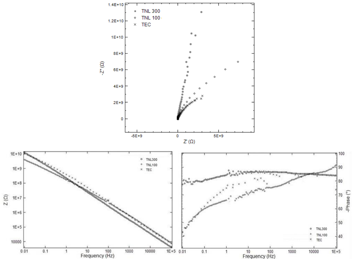
Figura 8. Impedância eletroquímica para solução de 40% (m/v) H 2 SO 4 . (a) Diagramas de Nyquist, (b) Módulo de Bode e (c) Ângulo de fase de Bode
