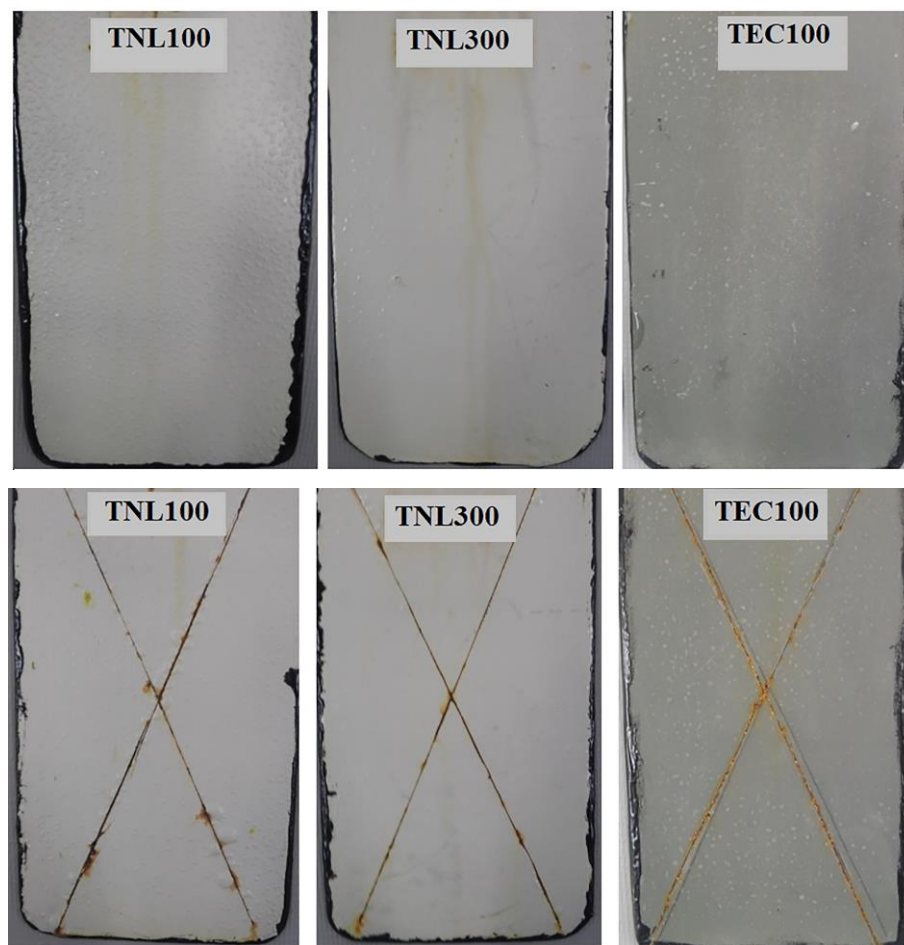
Figura 31 - Resultados do ensaio 100% umidade após 3500 h, sem e com incisão
