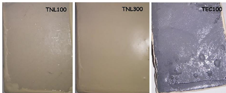
Figura 53. Corpos de provas após imersão na solução de 40% (m/v) H 2 SO 4
