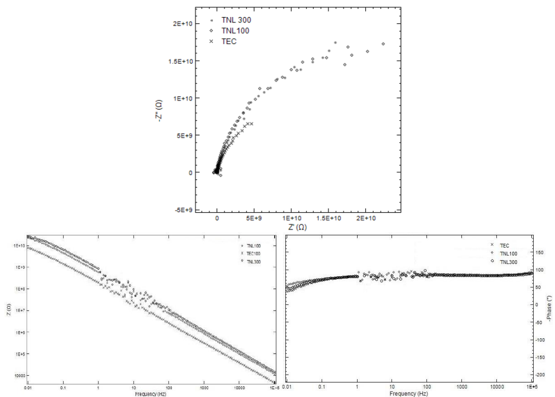
Figura 9. Impedância eletroquímica para solução de 3,5% (m/v) NaCl. (a) Diagramas de Nyquist, (b) Módulo de Bode e (c) Ângulo de fase de Bode
